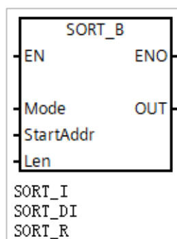
图 5 数组排序指令
